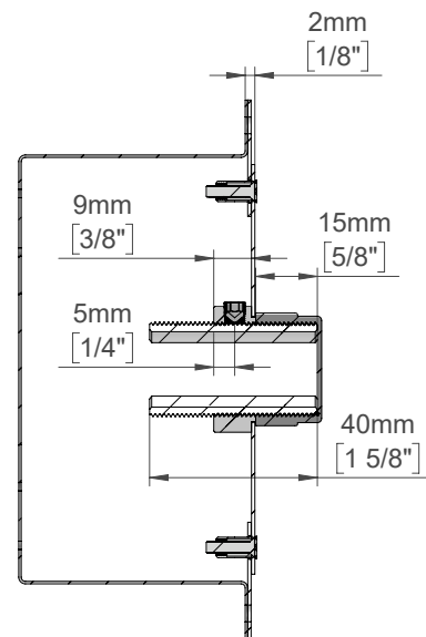
SEZIONE A-A SCALA 1 : 2
